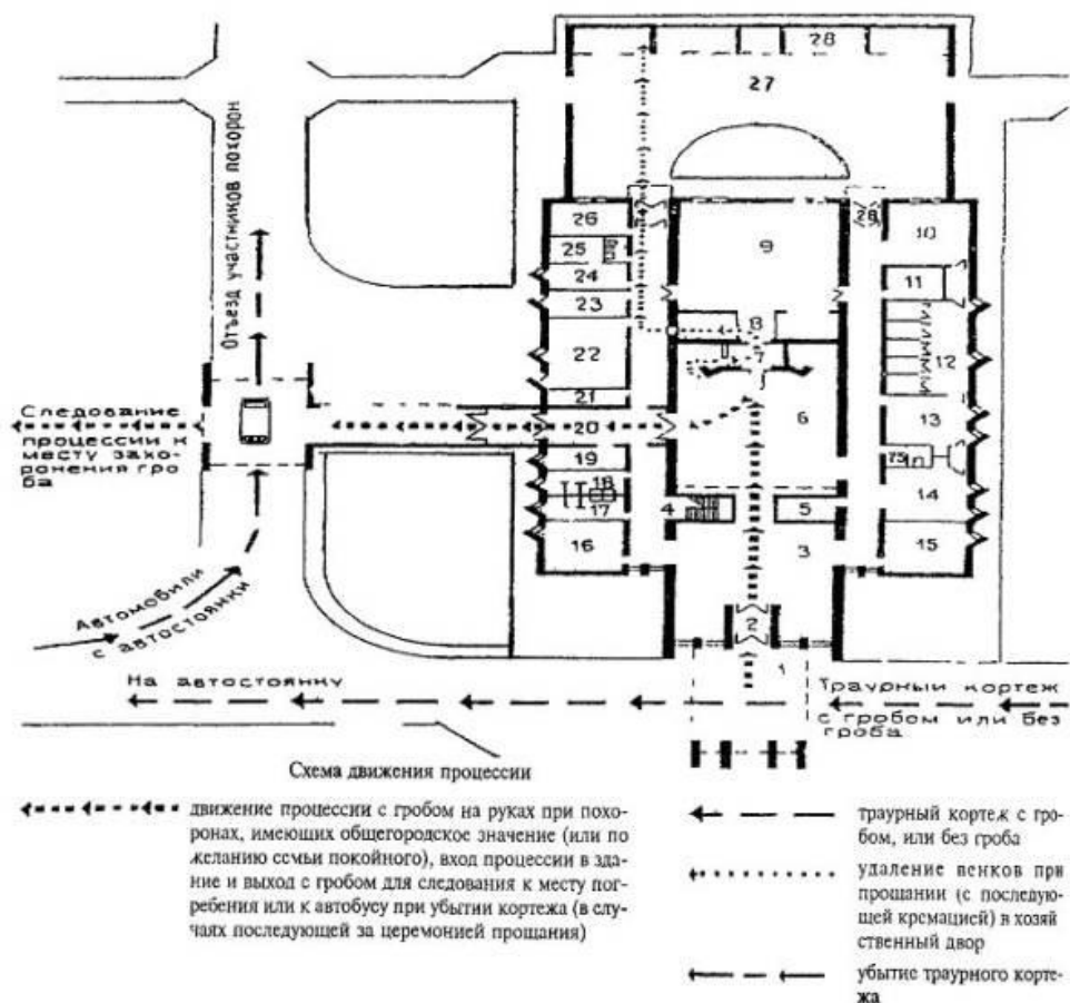
1 - козырек-навес главного входа, 2 - тамбур, 3 - зал ожидания, 4 - лестница на антресоль, 5 - комната формирования почетного караула, 6 - траурный зал, 7, 8 - передаточная камера, 9 - кремационный зал, 10 - приемная регистратуры, 11 - машинное отделение холодильной установки, 12 - холодильная камера, 13 - комната подготовки умерших к обряду, 14 - комната родственников, 15 - комната руководителя обряда и оформления документов, 16 - курительная, 17 - туалет для мужчин, 18 - туалет для женщин, 19 - комната оказания медицинской помощи, 20 -
