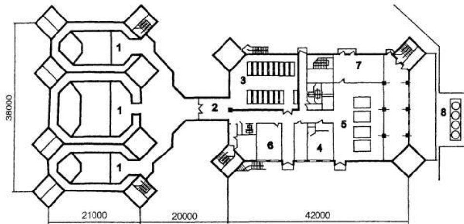
Рисунок 7 - Проект крематория в Ростове-на-Дону План на отм. 0,000
